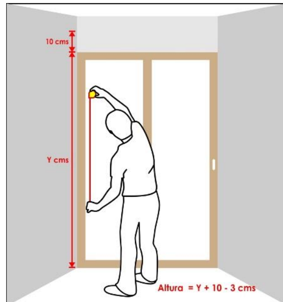
Altura: Ventana separada del techo
